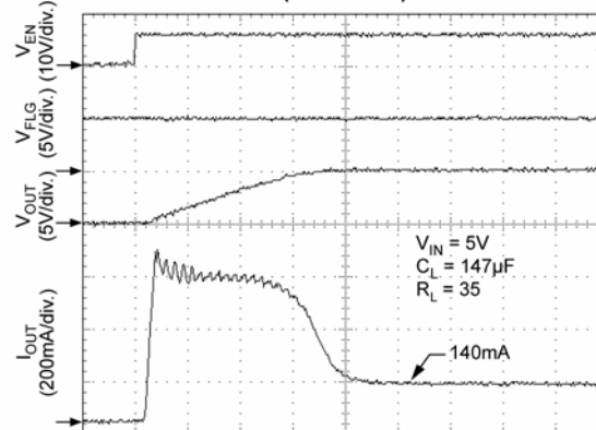
Turn-On (MIC2026-1)
