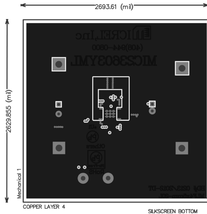
Bottom Layer
