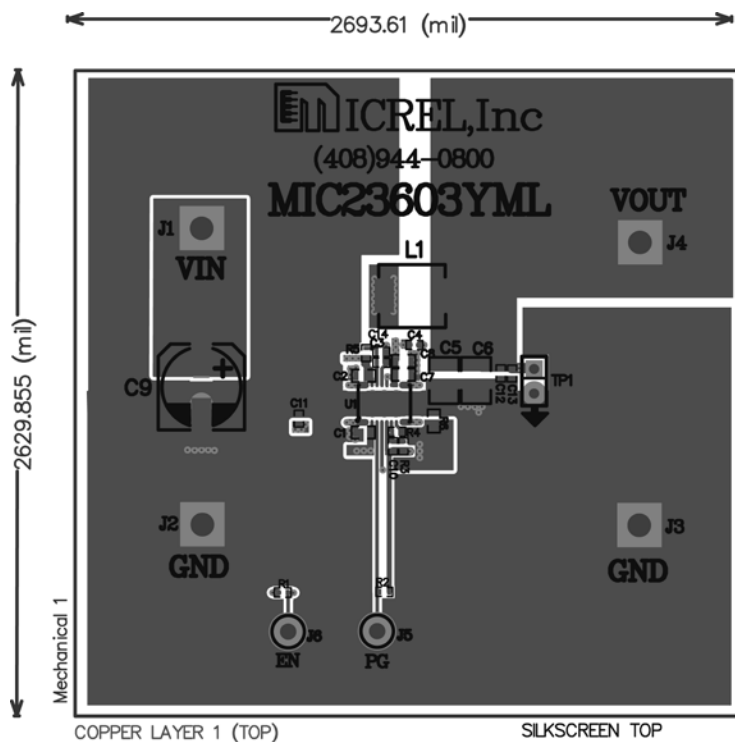
Top Layer
