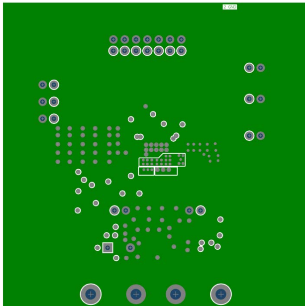
Copper Layer 2
