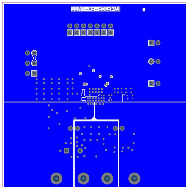
Bottom – Copper Layer 4
