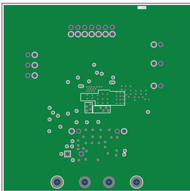
Copper Layer 2
