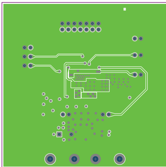
Copper Layer 3
