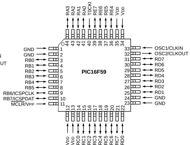
TQFP
