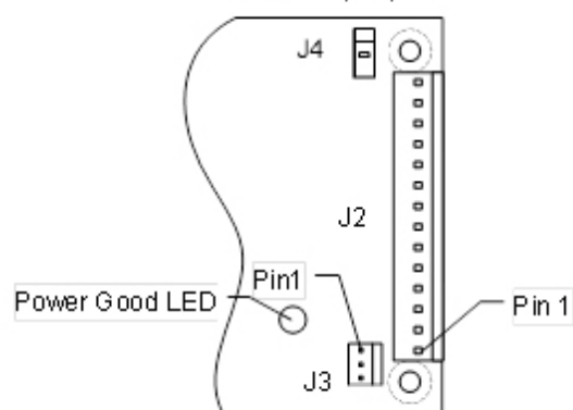
XR125-1, -7, -8
