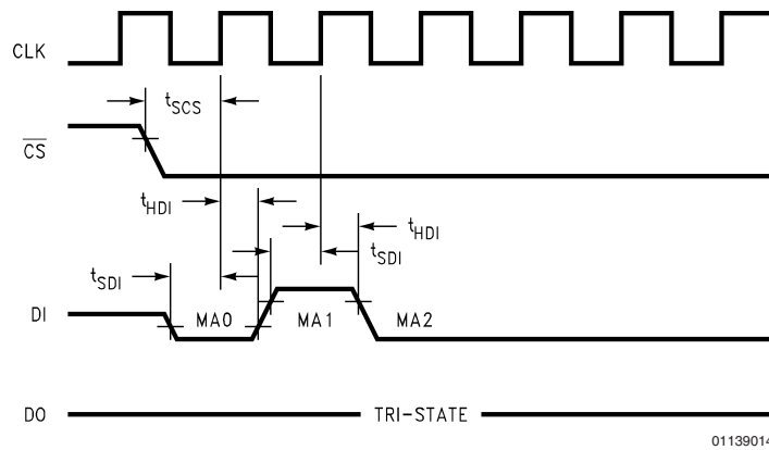
FIGURE 3. DI Timing
