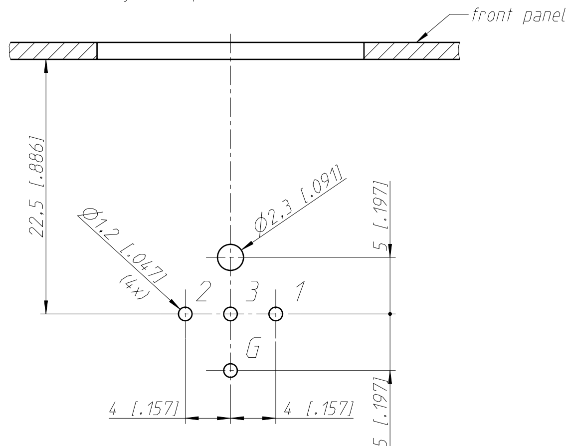
Print-Bohrplan (Bestückungsseite)
