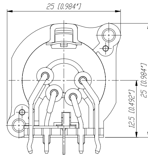
min. Einbauabstand min. assembling distance M 1:1
