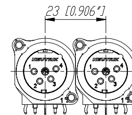
min. Einbauabstand min. assembling distance M 1:1
