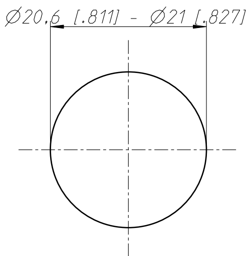
Frontplattenausschnitt Panel cut out
