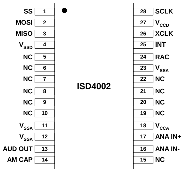
SOIC / PDIP
