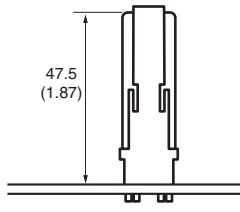
G2R-□7P
