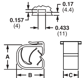
Edge Mount HCME06A12
