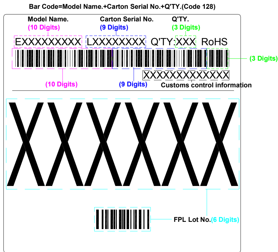
Carton Label
