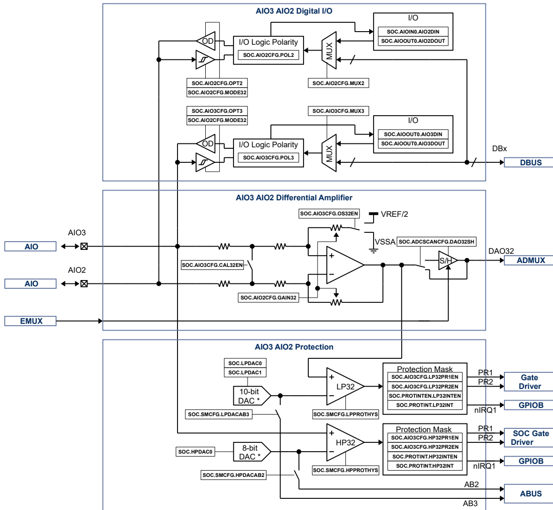
Figure 23-3. AIO3, AIO2
