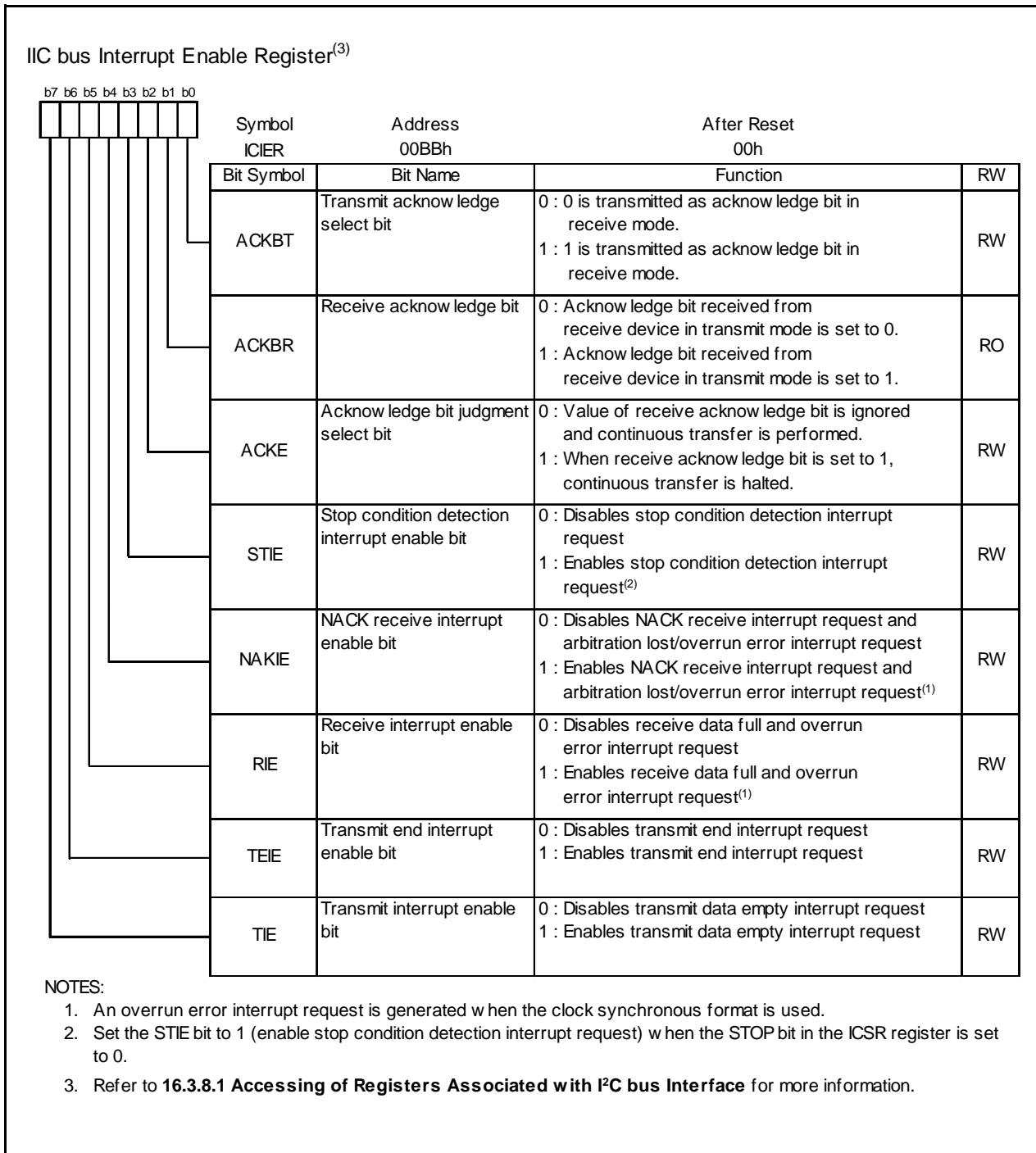
Figure 16.27 ICIER Register
