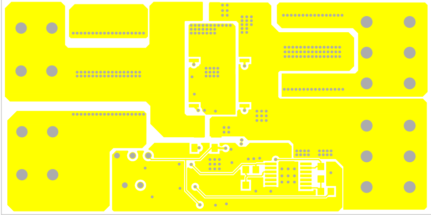
FIGURE 28. BOTTOM LAYER
