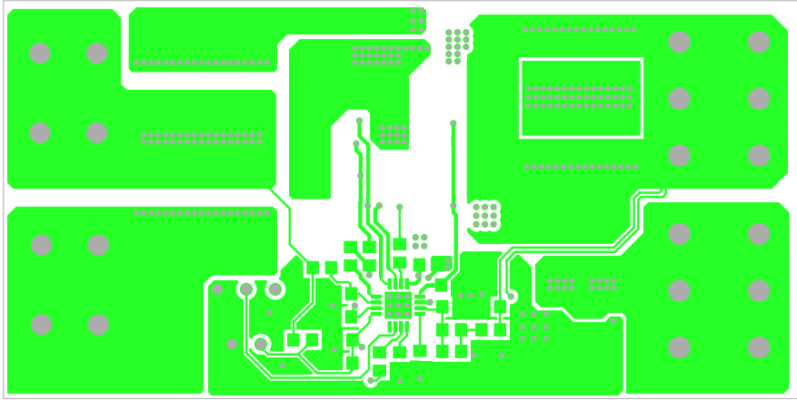
FIGURE 25. TOP LAYER
