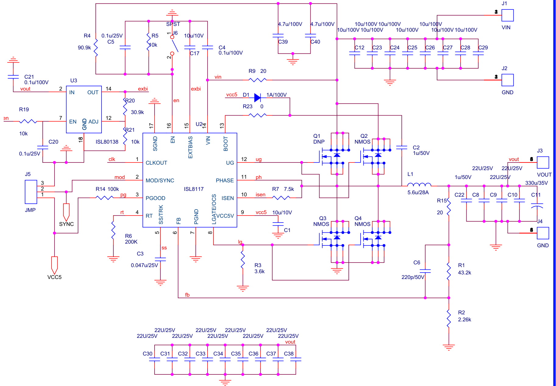
FIGURE 24. ISL8117DEMO2Z SCHEMATIC
