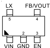
SOT-23-5/TSOT-23-5
