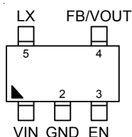
SOT-23-5/TSOT-23-5
