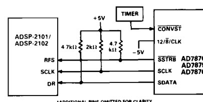
Figure 24. ADSP-2101/ADSP-2102 Serial Interface
