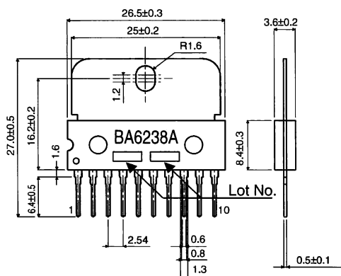
HSIP10 (Unit:mm)
