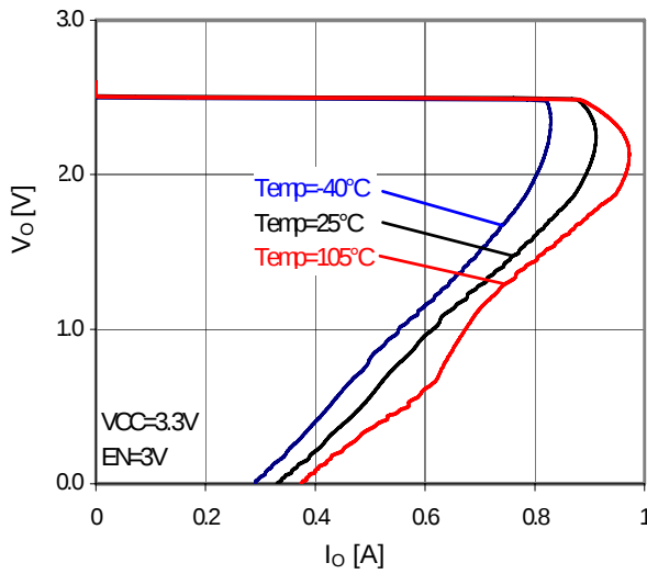
Fig.29 OCP
