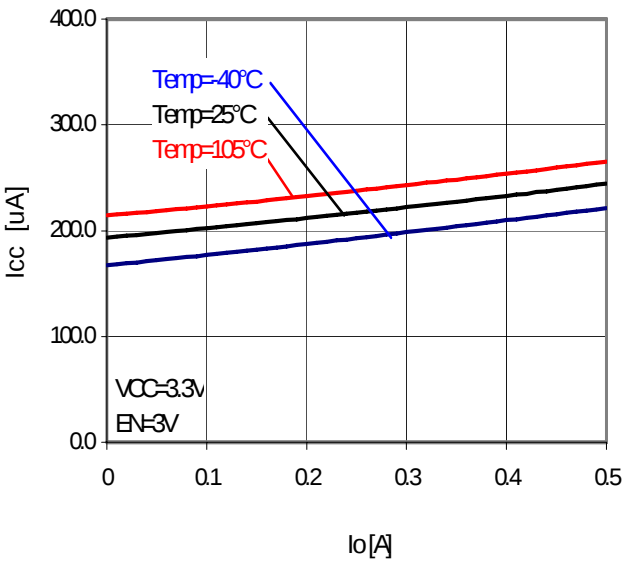
Fig.30 I_o-I_{cc}
