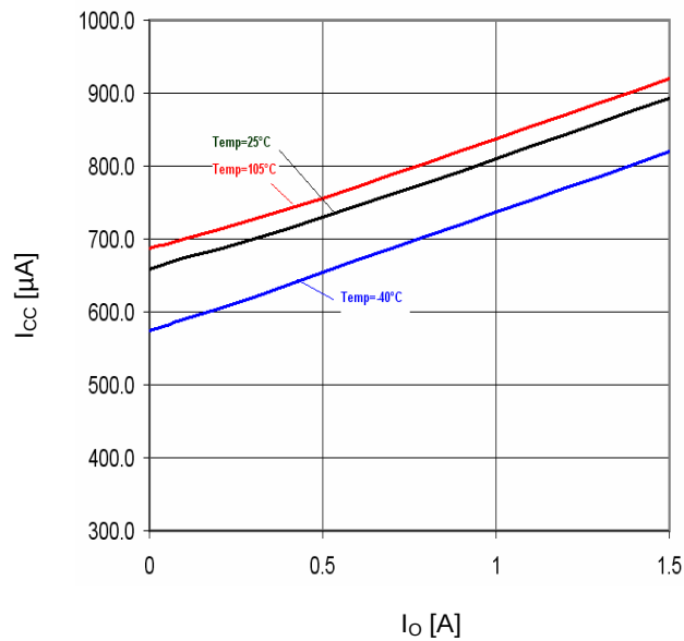
Fig.32 I_O - I_{CC}
