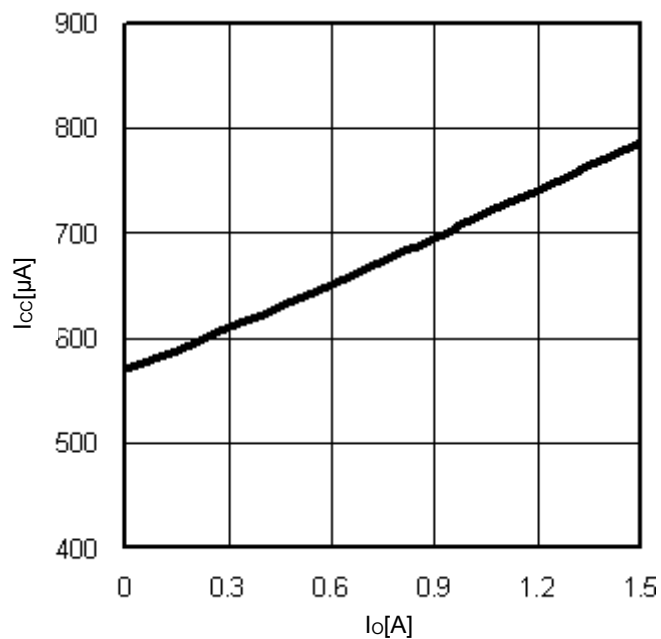
Fig.20 I_o - I_{cc}
