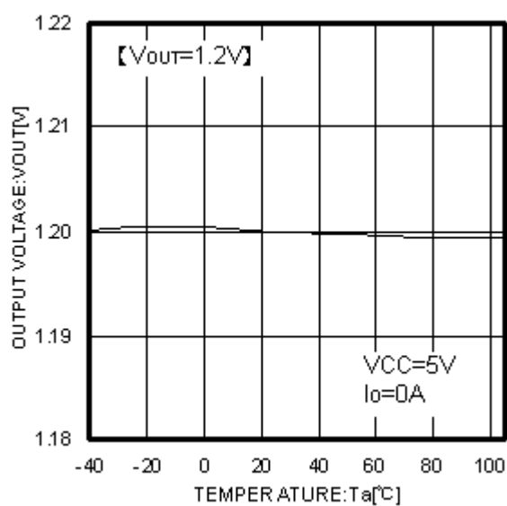
Fig.7 Ta - VOUT
