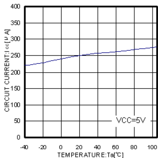
Fig.12 T_a - I_{cc}
