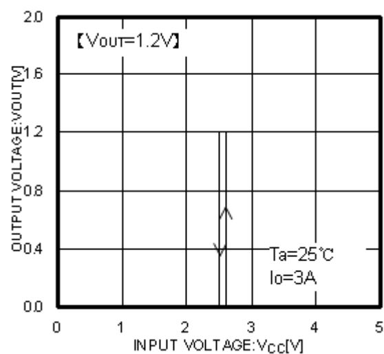
Fig.4 Vcc - VOUT
