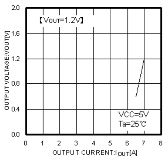
Fig.6 IOUT - VOUT
