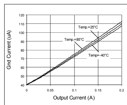
Fig. 126 IOOUT - IGND
