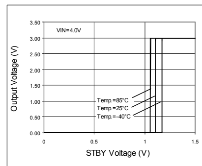
Fig. 129 STBY Threshold
