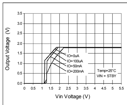
Fig. 34 Output Voltage
