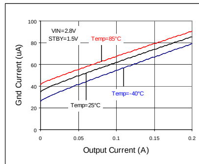
Fig 7. IOUT - IGDND
