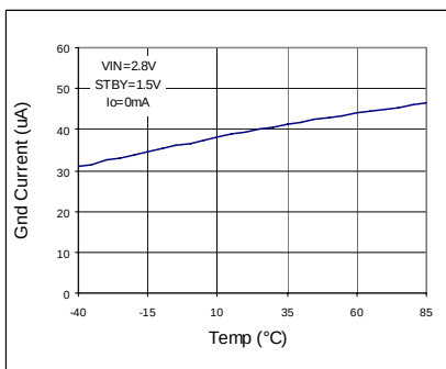
Fig 12. IGDND - Temp
