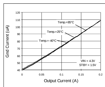
Fig. 155 IOUT - IIGN
