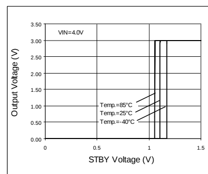
Fig. 129 STBY Threshold
