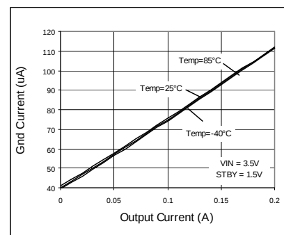
Fig. 10 IOU - IGD
