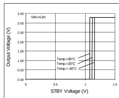
Fig. 158 STBY Threshold
