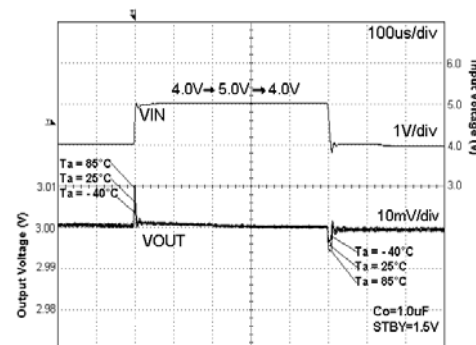
Fig. 149 VIN Response I_{out} = 10\text{mA}
