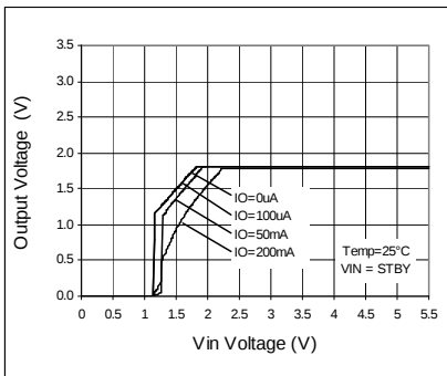
Fig. 34 Output Voltage
