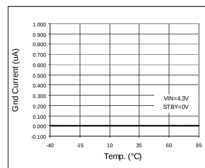
Fig. 161 IIGN vs Temp (STBY)
