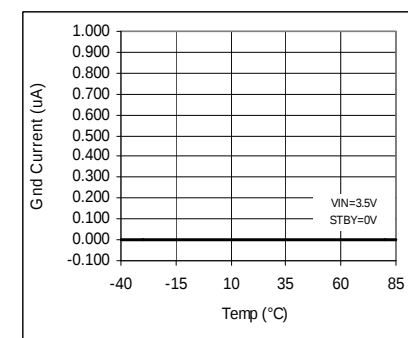
Fig. 16 IGD vs. Temp (STBY)
