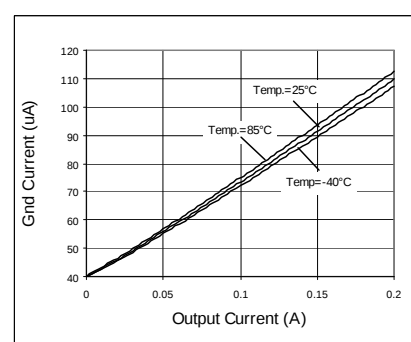
Fig. 126 IOUT - IIGN
