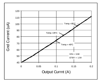
Fig. 97 IOUT - IGND
