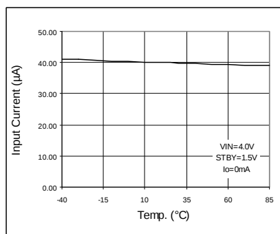
Fig. 131 IIGN vs Temp
