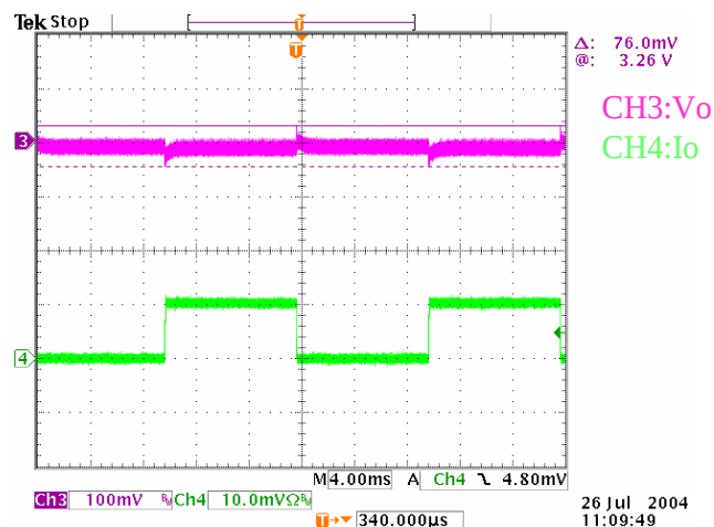
Transient response(0-5A).
