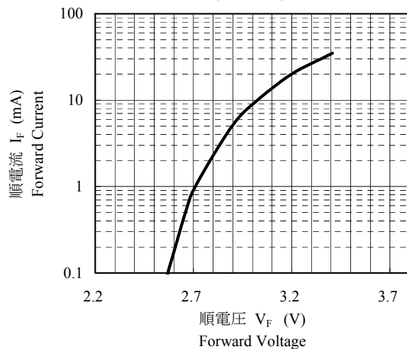
順電流 — 順電圧特性 Forward Current vs. Forward Voltage ( T_c=25\text{ }^{\circ}\text{C} )
