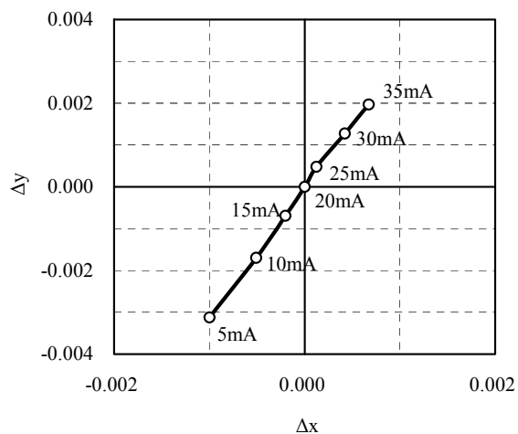
色度座標 — 順電流特性 Chromaticity coordinates vs. Forward Current ( T_c=25\text{ }^{\circ}\text{C} )
