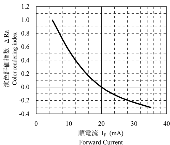
演色評価指数 — 順電流特性 Color rendering index vs. Forward Current ( T_c=25\text{ }^{\circ}\text{C} )
