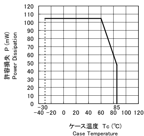
許容損失低減曲線 Power Dissipation Derating Curve
