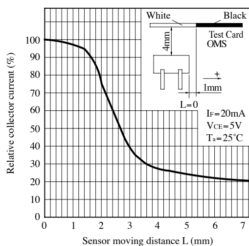
Fig.10 検出位置特性 (1)
