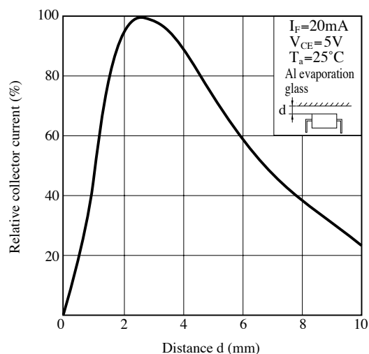
Fig.12 相对光電流—距離特性 (参考値)
