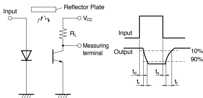
Fig.9 応答時間の測定回路
