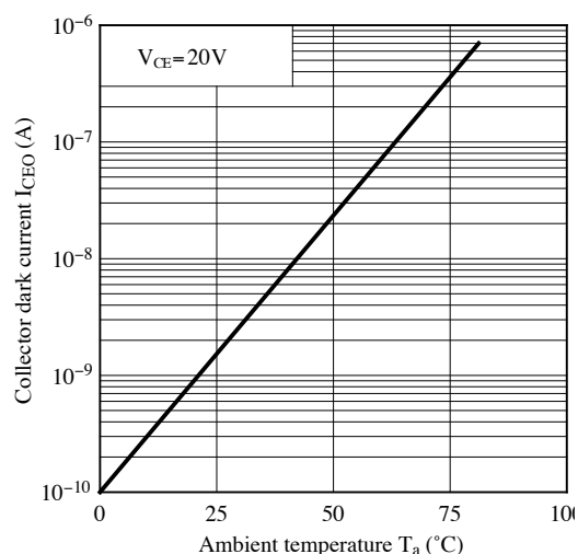
Fig.7 暗電流—周囲温度特性
