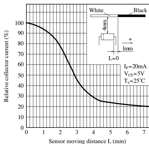
Fig.11 検出位置特性 (2)
