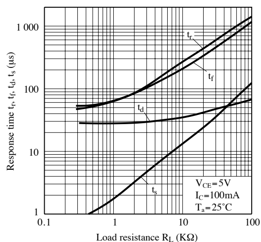
Fig.8 応答時間—負荷抵抗特性
