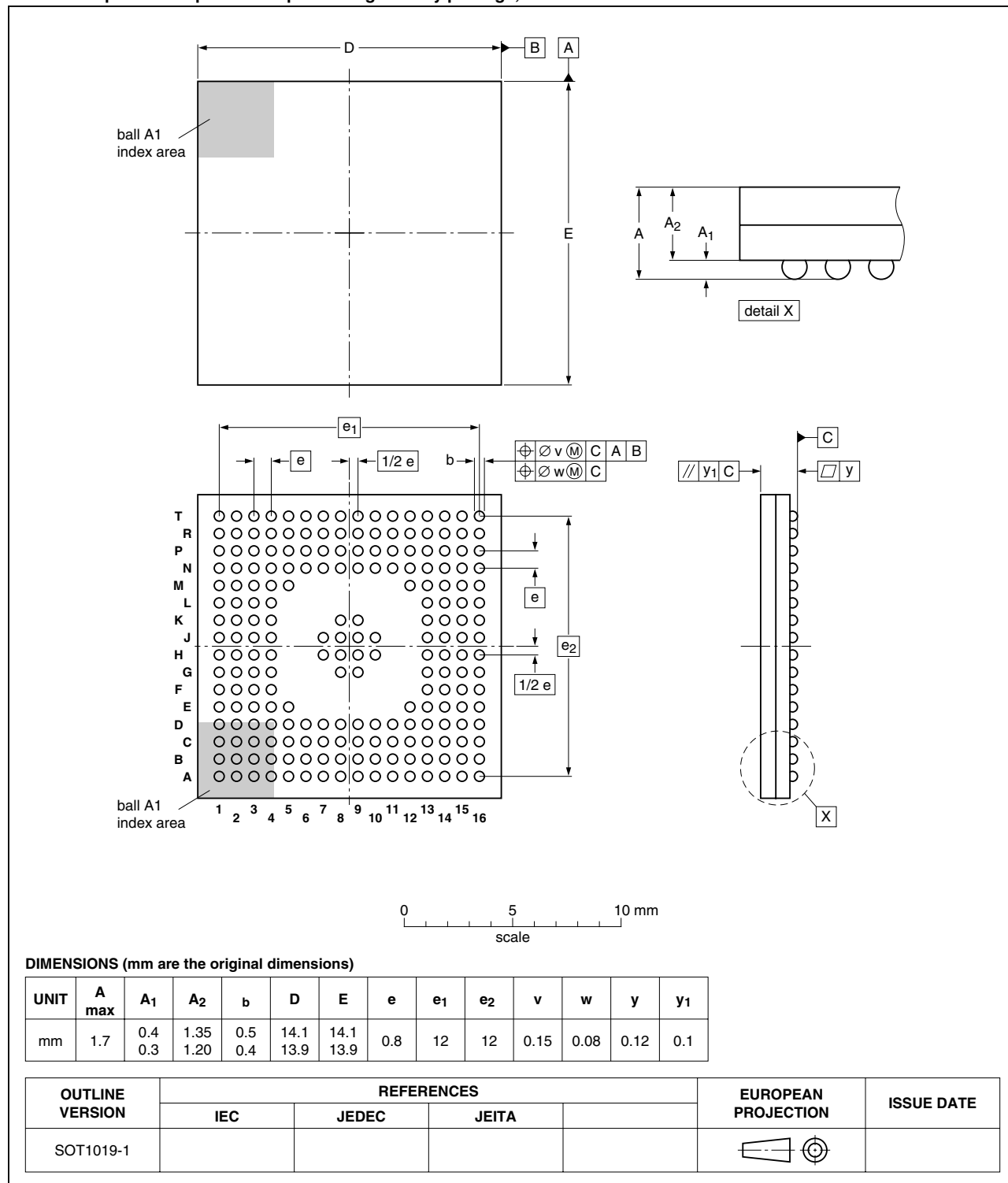
SOT1019-1
