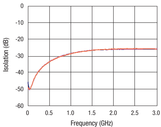
RF1 to RF3 Isolation
