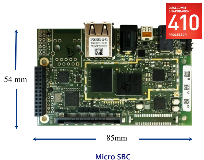
Micro SBC
