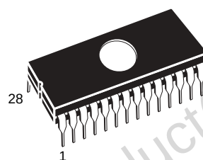
FDIP28W (F)
