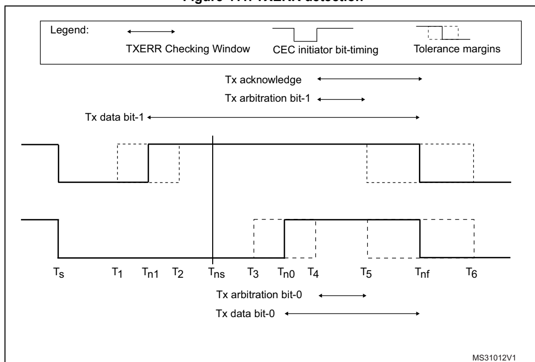
Figure 411. TXERR detection
