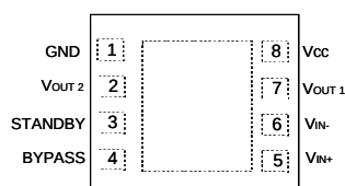
TS421IDT: SO8 TS421IST, TS421-xIST: MiniSO8
