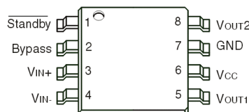
TS421IQT, TS421-xIQT: DFN8
