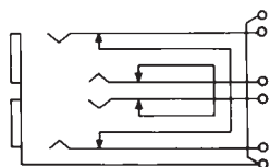
TT89 SCHEMATIC
