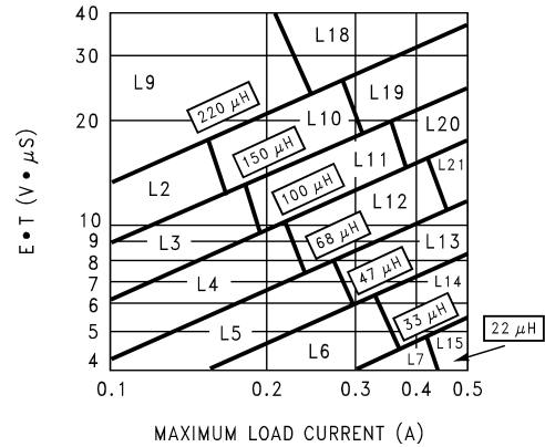
Figure 27. LM2671-ADJ
