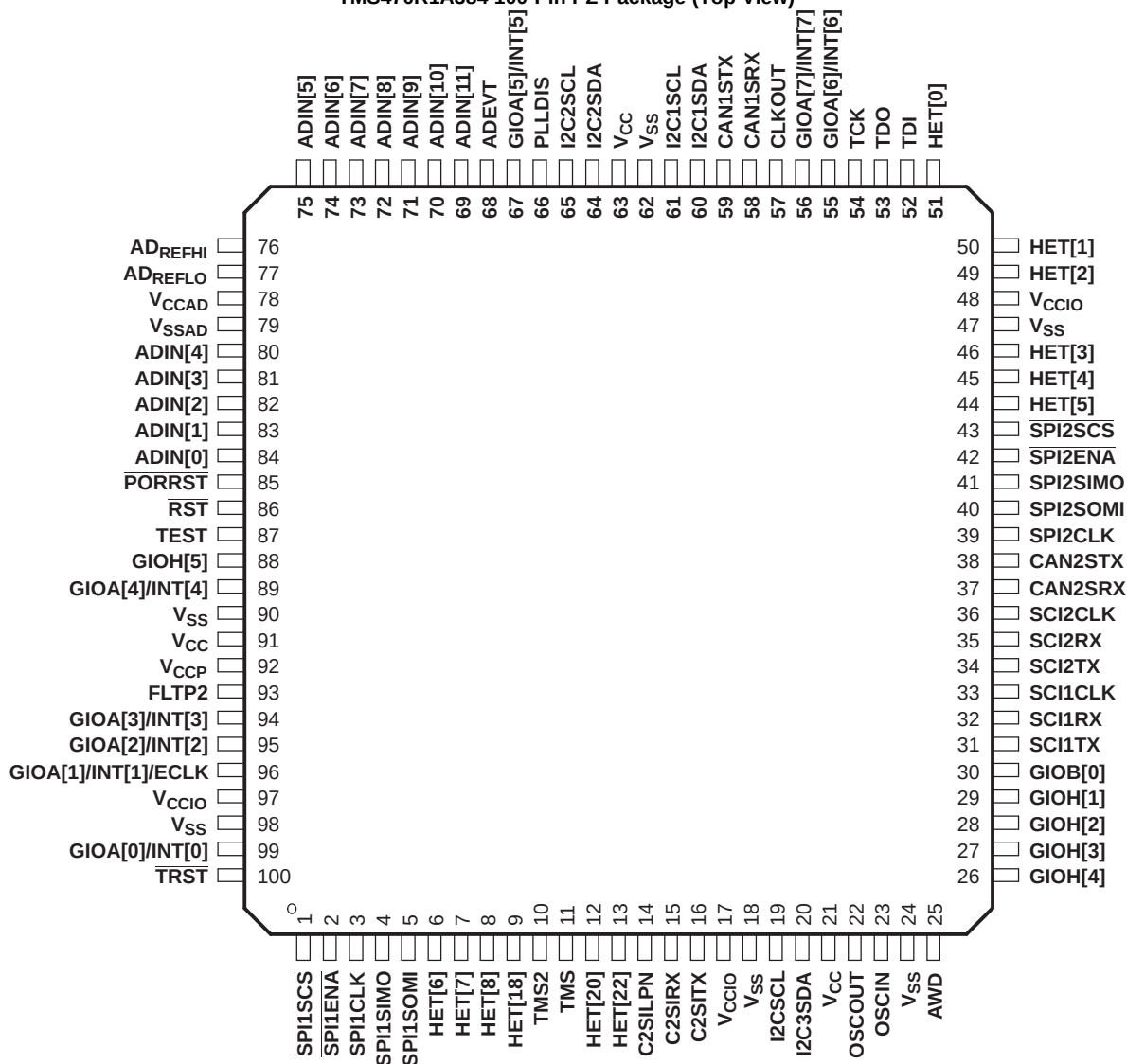
TMS470R1A384 100-Pin PZ Package (Top View)
