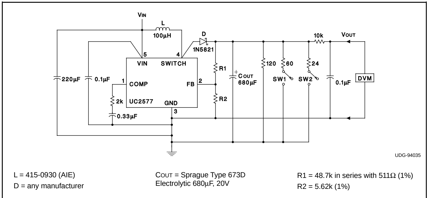
Figure 1. Circuit Used to Specify System Parameters
