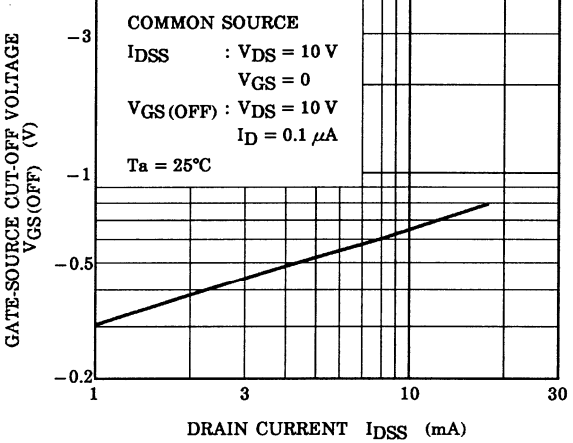
V_{GS}(\text{OFF}) - I_{DSS}
