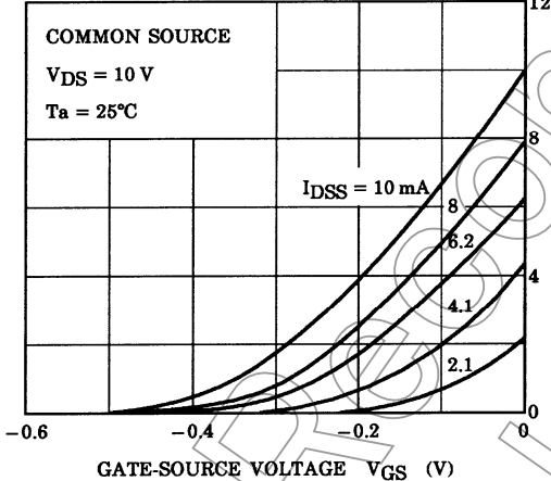
I_D - V_{GS}
