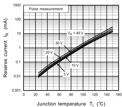
Fig. 10.8 I_R - T_j
