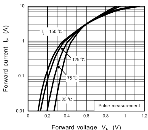
Fig. 10.1 I_F - V_F
