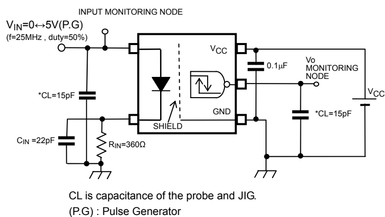
TEST CIRCUIT 5 : t_{pHL} , t_{pLH}
