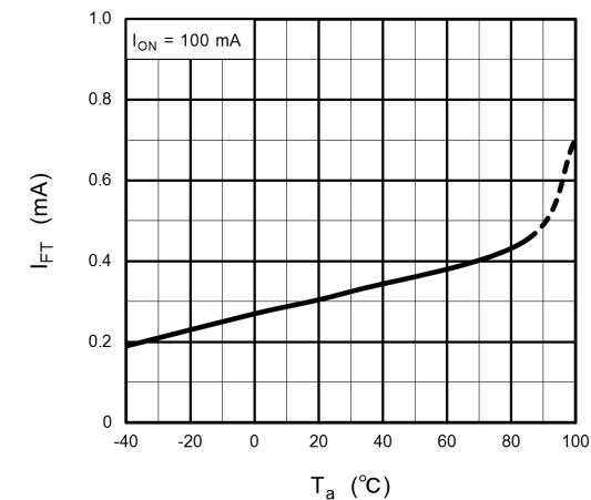
Fig. 12.1.6 I_{FT} - T_a
