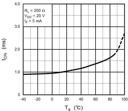
Fig. 12.1.7 t_{ON} - T_a
