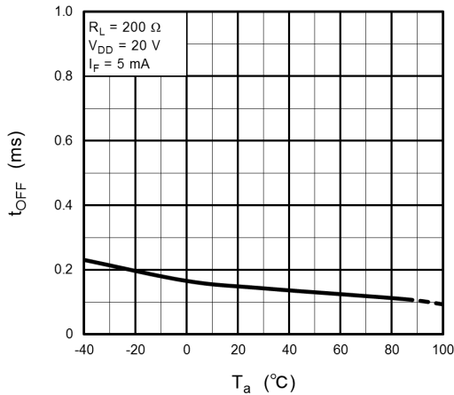
Fig. 12.1.8 t_{OFF} - T_a
