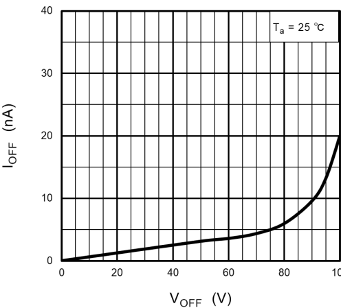
Fig. 12.1.10 I_{OFF} - V_{OFF}
