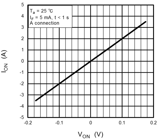
Fig. 13.1.4 I_{ON} - V_{ON}
