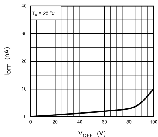
Fig. 13.1.10 I_{OFF} - V_{OFF}
