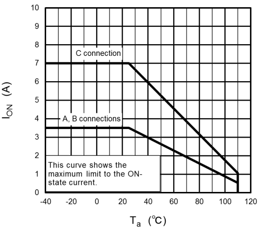
Fig. 13.1.2 I_{ON} - T_a
