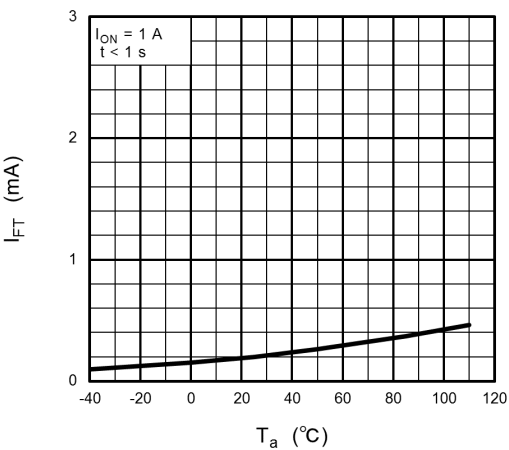
Fig. 13.1.6 I_{FT} - T_a
