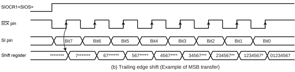
Figure 10-4 Shift Edge
