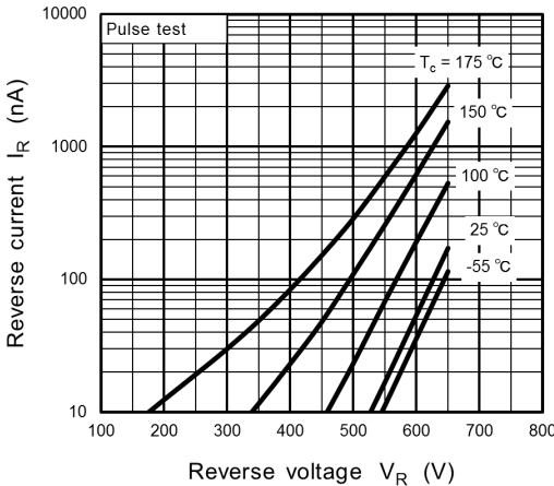
Fig. 9.3 I_R - V_R
