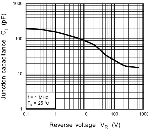
Fig. 9.4 C_j - V_R
